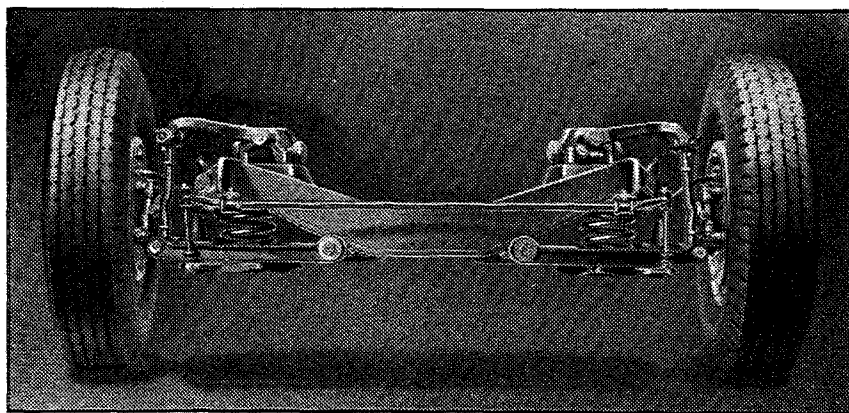
Cadillac '61'-LaSalle Knee Action
